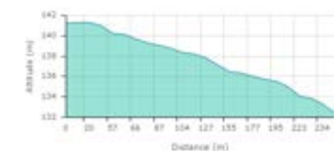
PROFIL ALTIMÉTRIQUE
