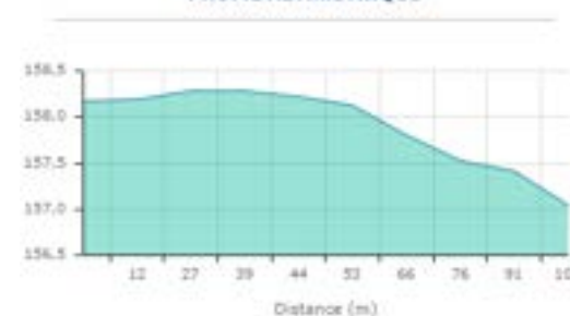
PROFIL ALTIMÉTRIQUE
