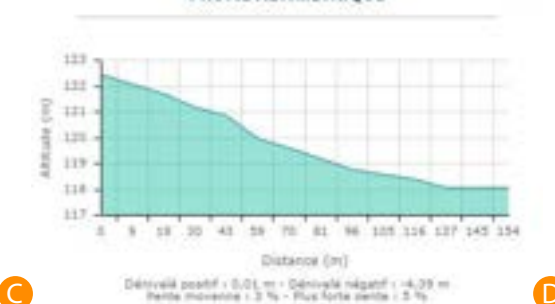
PROFIL ALTIMÉTRIQUE
