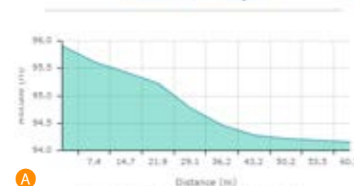
PROFIL ALTIMÉTRIQUE
