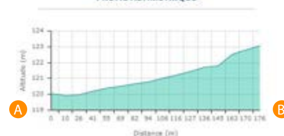
PROFIL ALTIMÉTRIQUE
