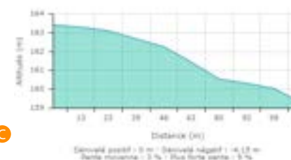
PROFIL ALTIMÉTRIQUE
