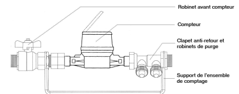
Schéma-type d'un ensemble de comptage
